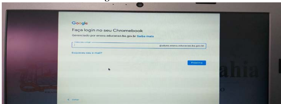
Figura 5 - Tela inicial
