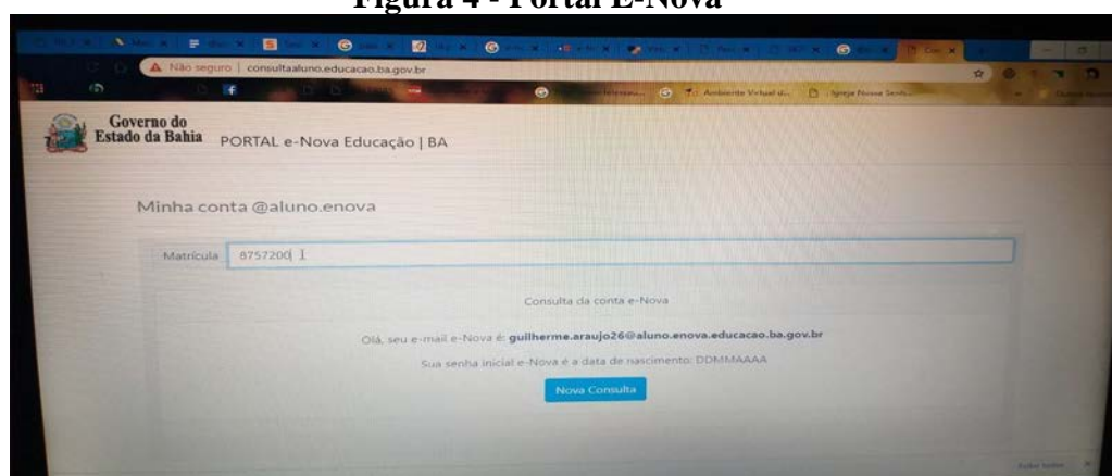
Figura 4 - Portal E-Nova
